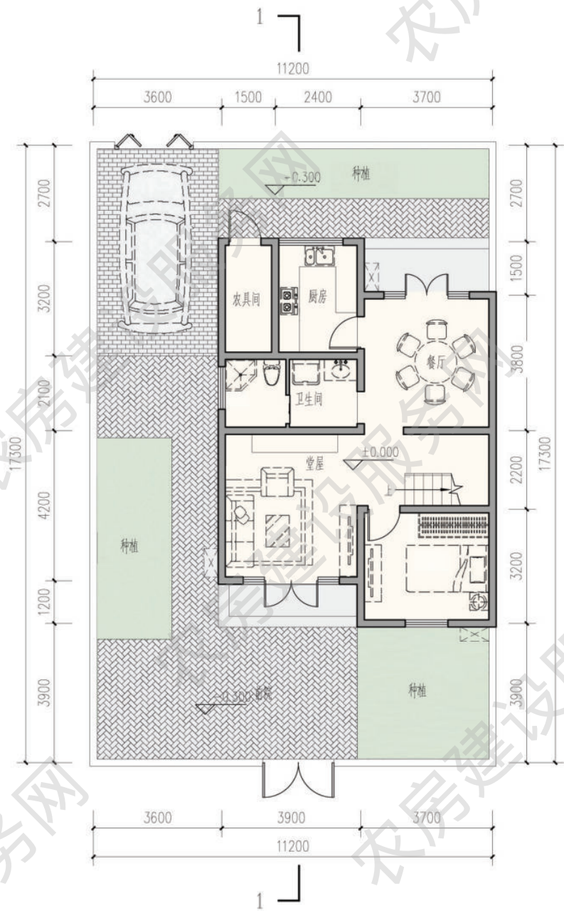
一层平面图 本层建筑面积 74 平方米
