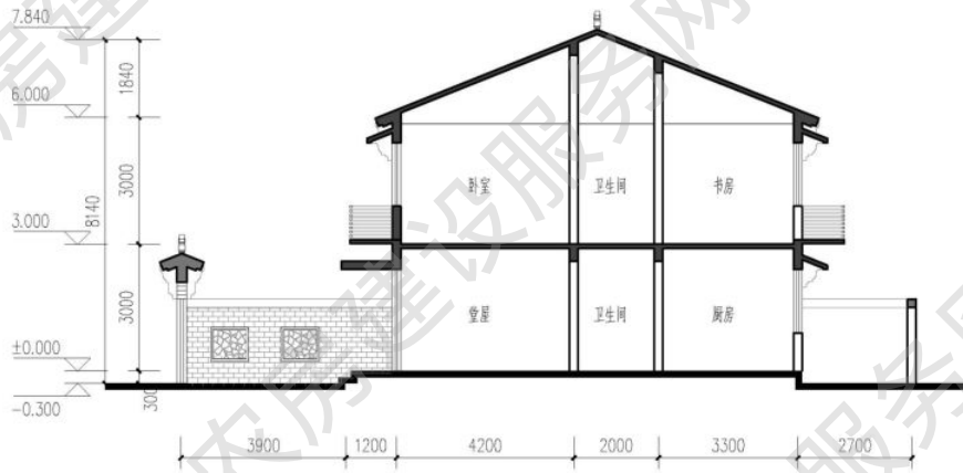
1-1 剖面图
