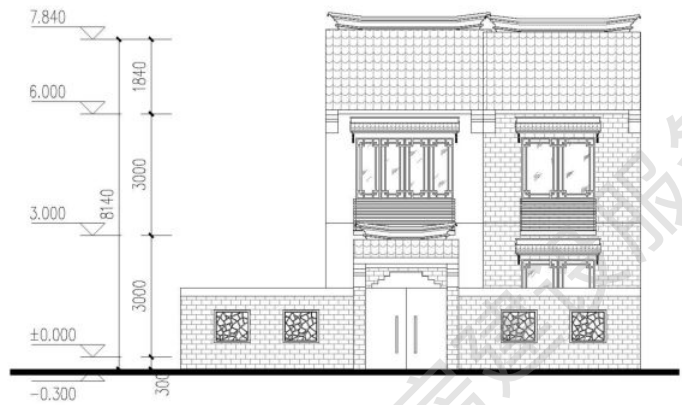
南立面图
