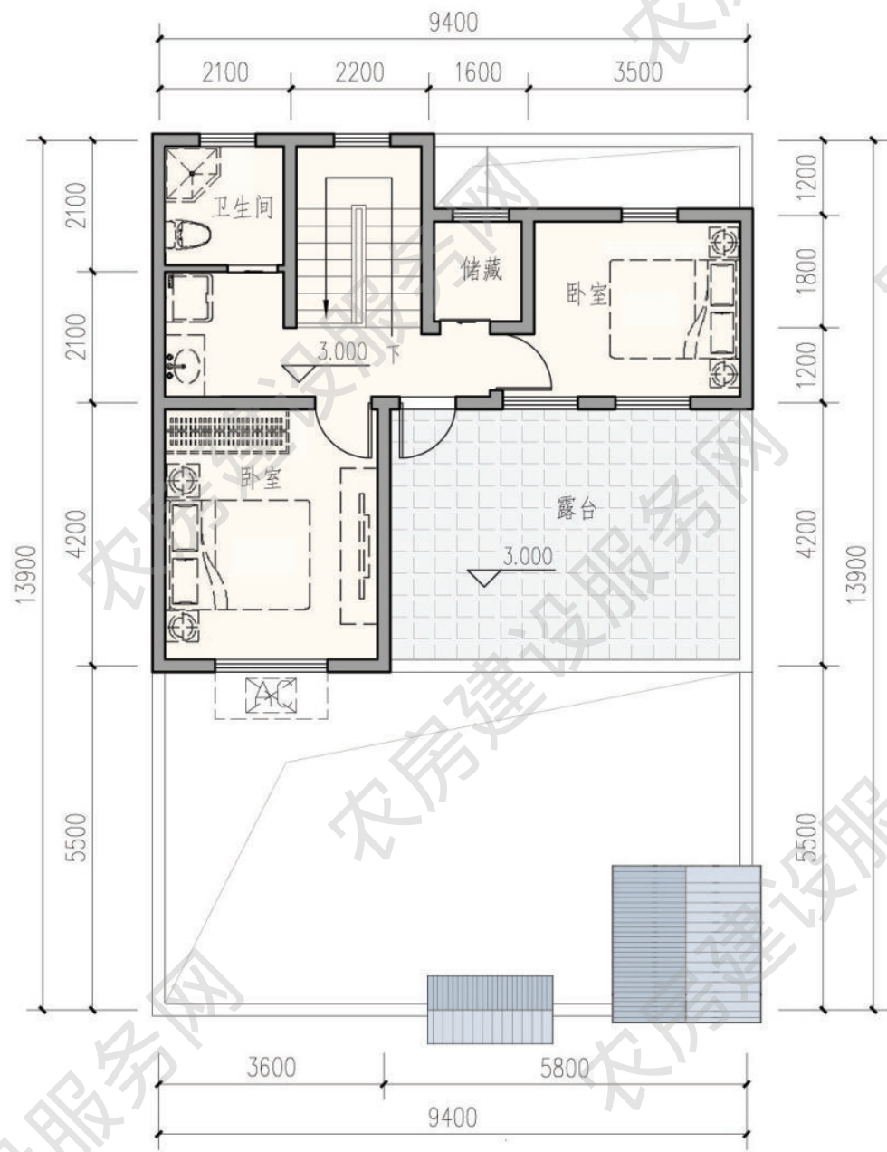
二层平面图 本层建筑面积 52 平方米
