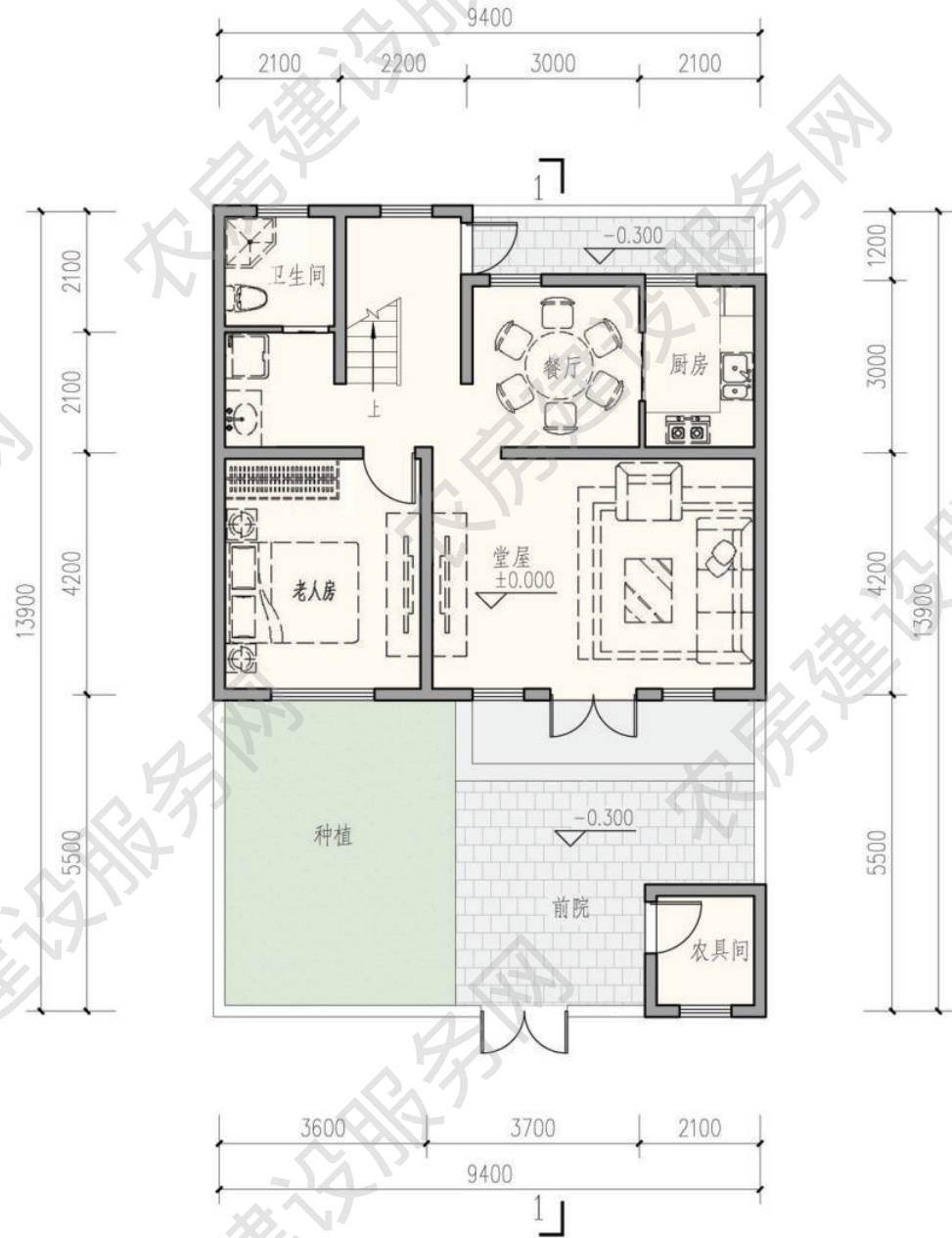
一层平面图 本层建筑面积 81 平方米
