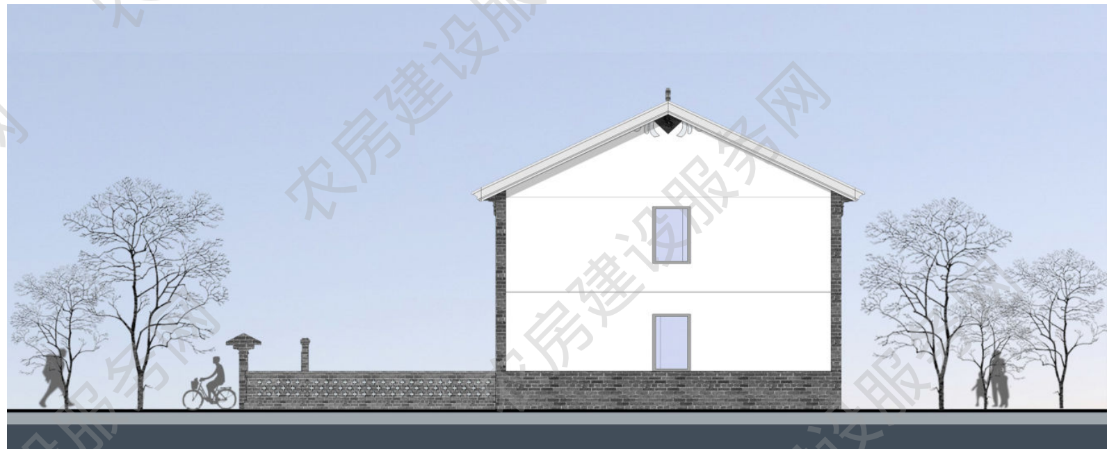
东立面图
