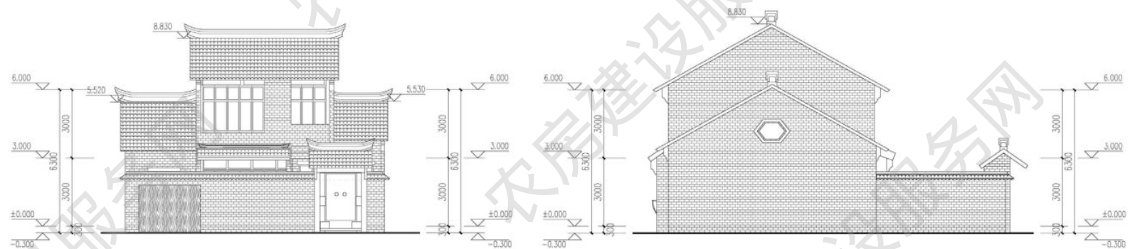
南立面图
