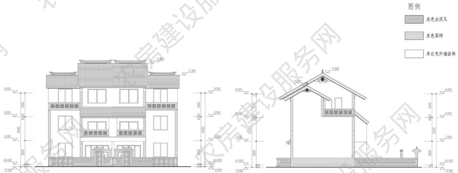
南立面图
