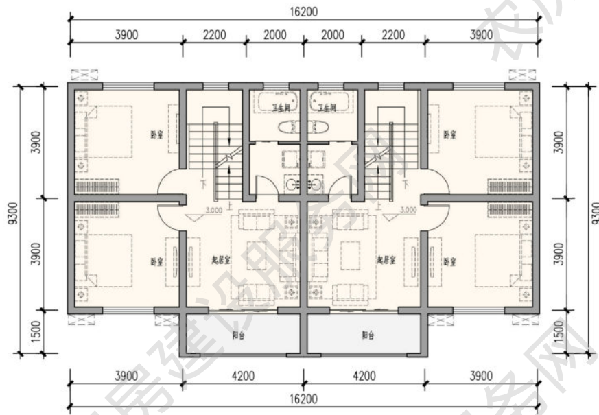
二层平面图 本层建筑面积 68.37 平方米
