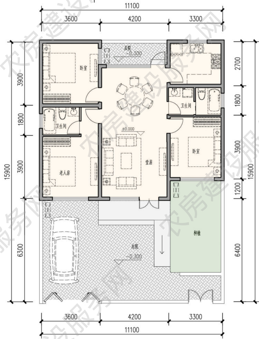
一层平面图 本层建筑面积 100.78 平方米
