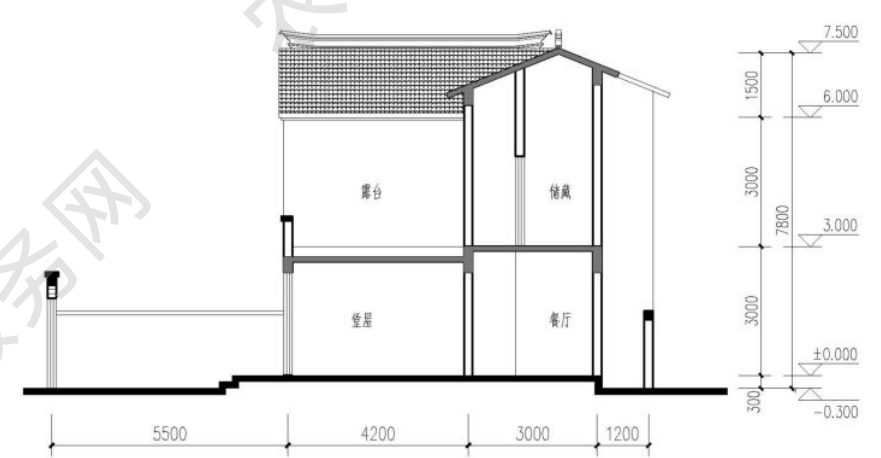
1-1 剖面图
