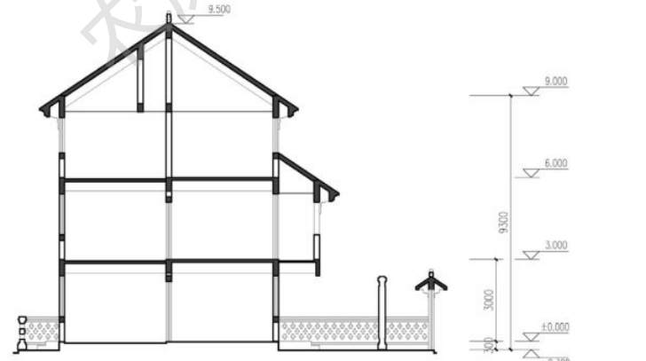
1-1 剖面图
