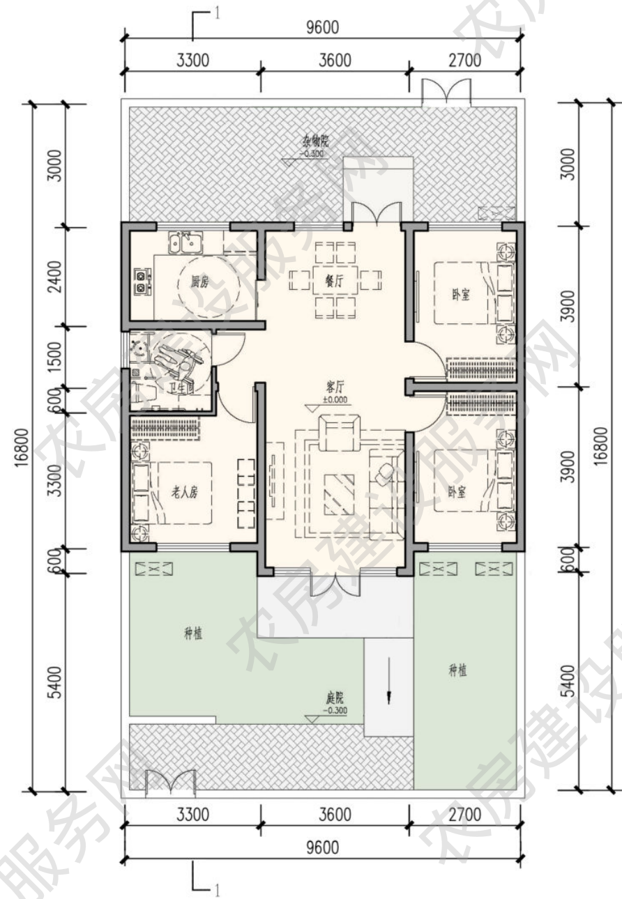
一层平面图 本层建筑面积 80.68 平方米
