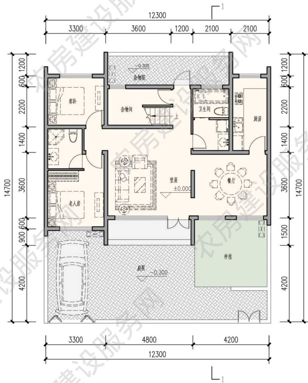
一层平面图 本层建筑面积 98.08 平方米
