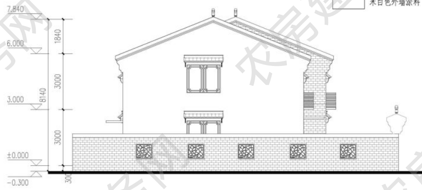
西立面图
